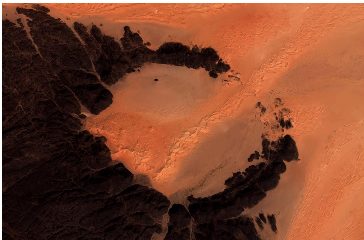
Pince de crabe d'Arakao (Niger - Aïr) : Image Sentinel 2 (ESA)
